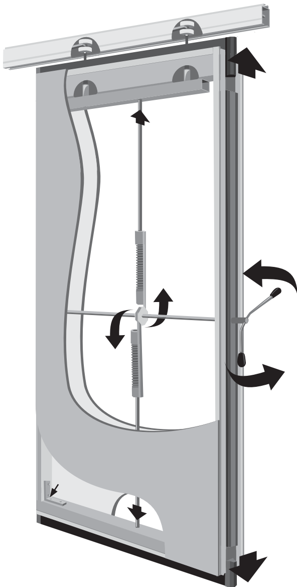
3-S-Verriegelungssystem
